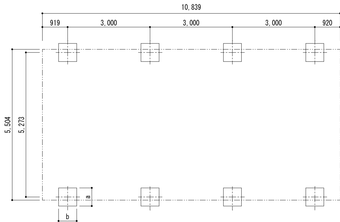
■基礎配置図
